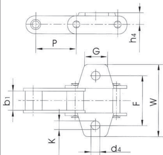
MOCOWANIE TYPU "K1"
