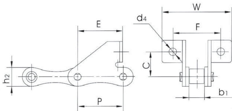
MOCOWANIE TYPU "F4"
